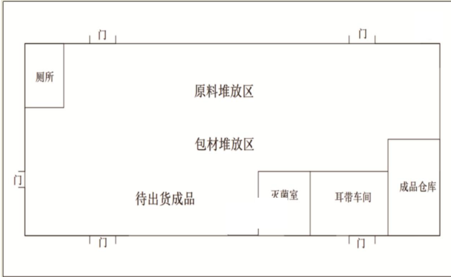
附图5 厂房1F平面布置图
