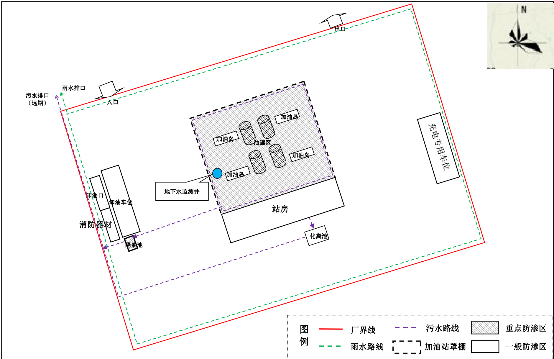
附图3 项目厂区平面布置图及雨污管网图
